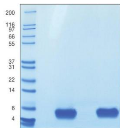
SDS-PAGE
